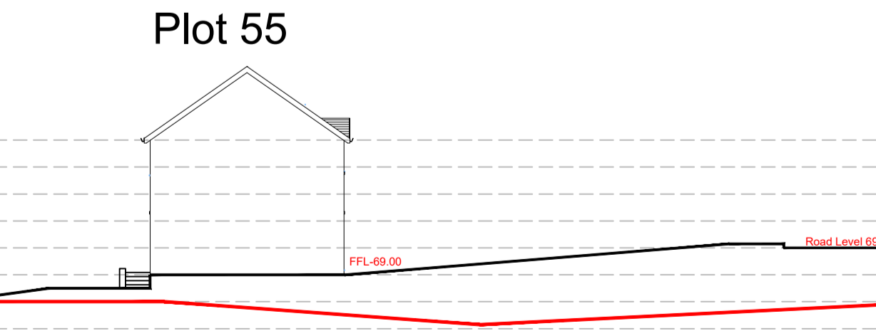
Section D:D 1:200
