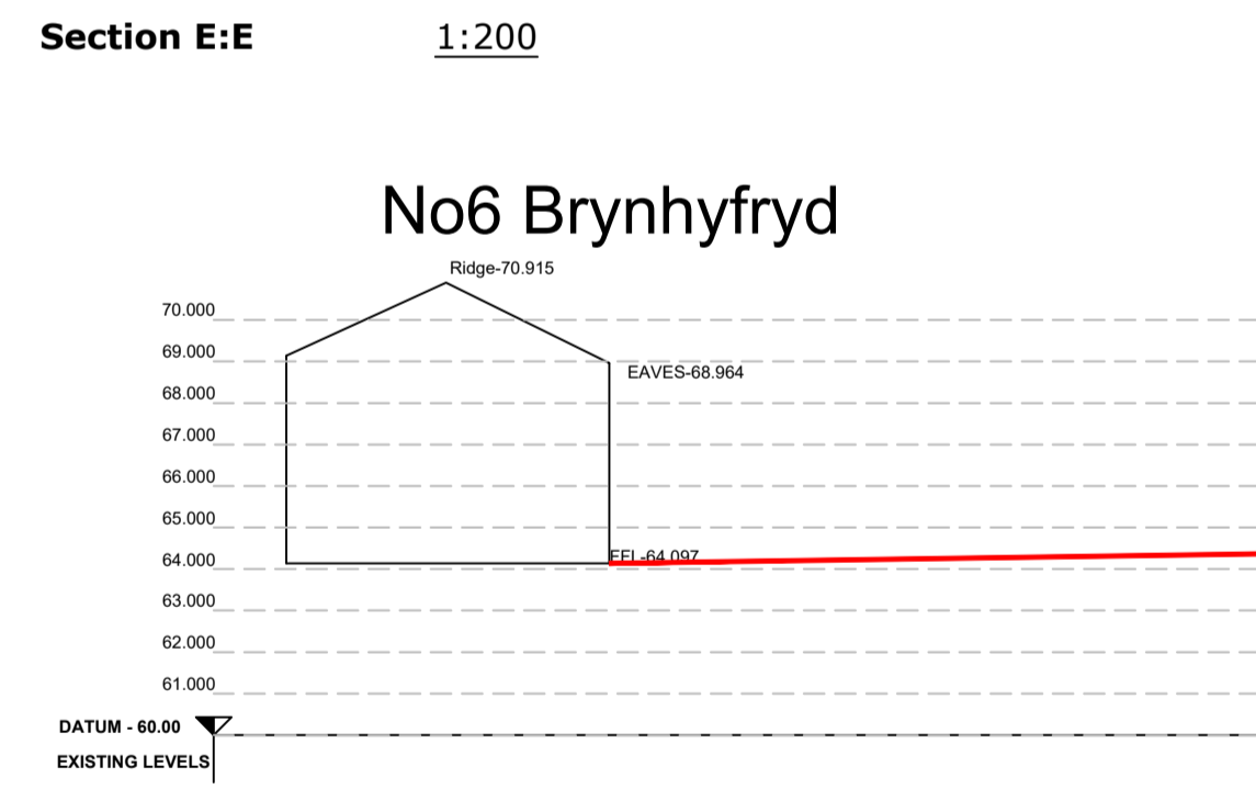
Section E:E 1:200
