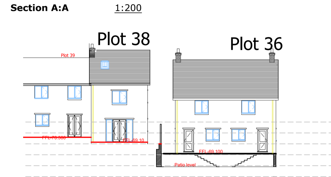
Section A:A 1:200
